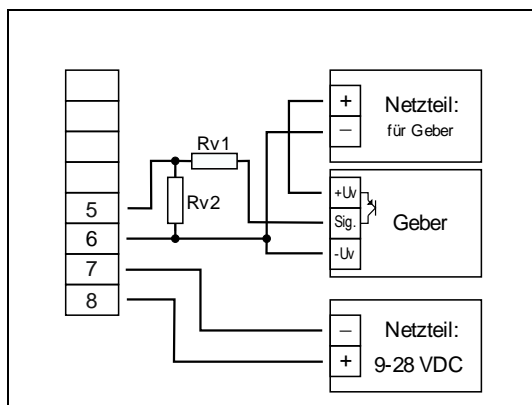
Anschluss eines Gebers (mit getr. Versorgung) mit PNP-Ausgang und externer Widerstandsbeschaltung
