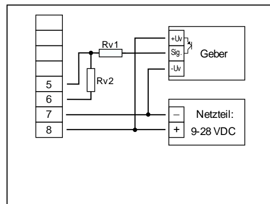
Anschluss eines Gebers (ohne eigene Versorgung) mit PNP-Ausgang und externer Widerstandsbeschaltung
