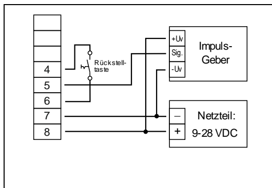
manuelles Rücksetzen mit externem Taster
