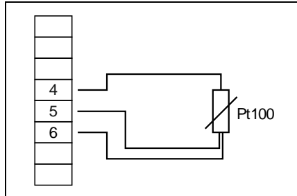
Pt100-Temperaturfühler (3-Leiter)
