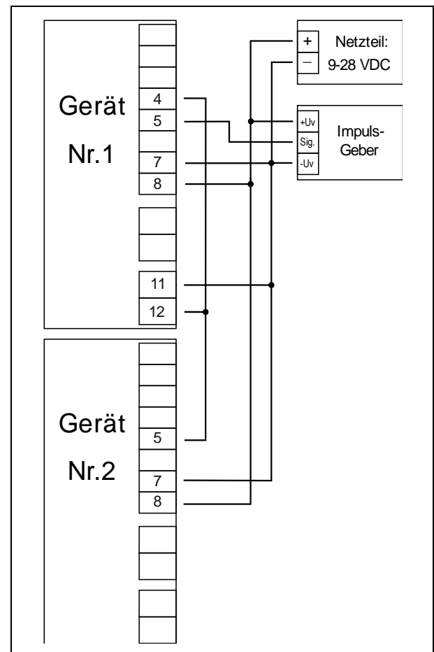
GIR 300 kaskadierend
