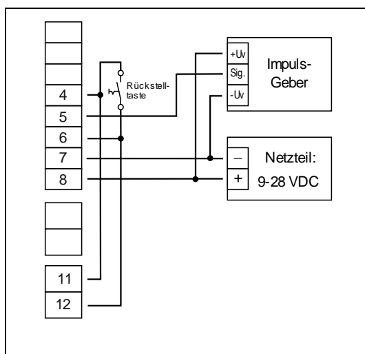
automatisches Rücksetzen mit Ausgang 1 und zusätzliches man. Rücksetzen mit externem Taster Anschlussshinweis: Ausgang 2 darf auch nur noch Kleinspannungen schalten!
