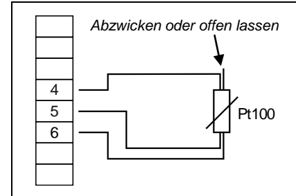
Pt100-Temperaturfühler (4-Leiter)
