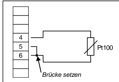
Pt100-Temperaturfühler (2-Leiter)
