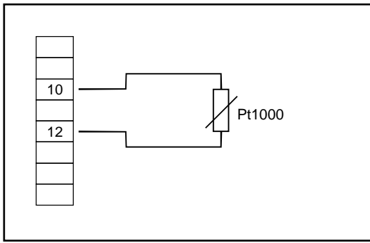
Pt1000-Temperaturfühler (2-Leiter)
