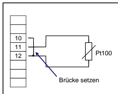
Pt100-Temperaturfühler (2-Leiter)
