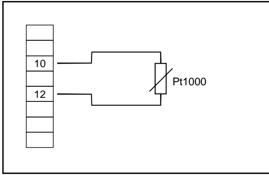
Pt1000-Temperaturfühler (2-Leiter)
