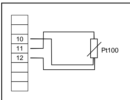
Pt100-Temperaturfühler (3-Leiter)
