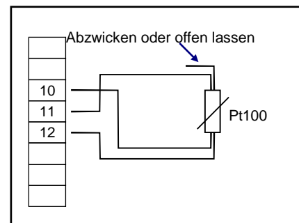
Pt100-Temperaturfühler (4-Leiter)
