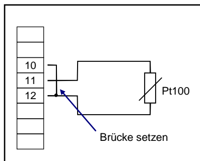
Pt100-Temperaturfühler (2-Leiter)
